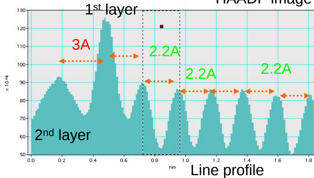
HAADF image
