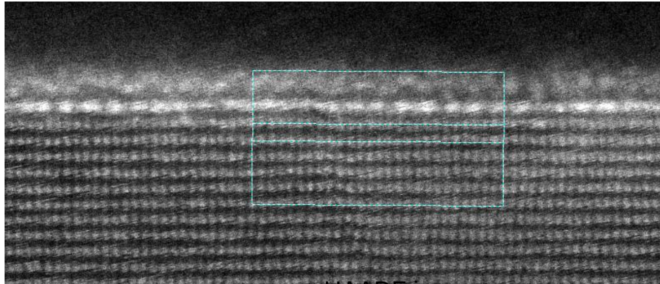
HAADF image
